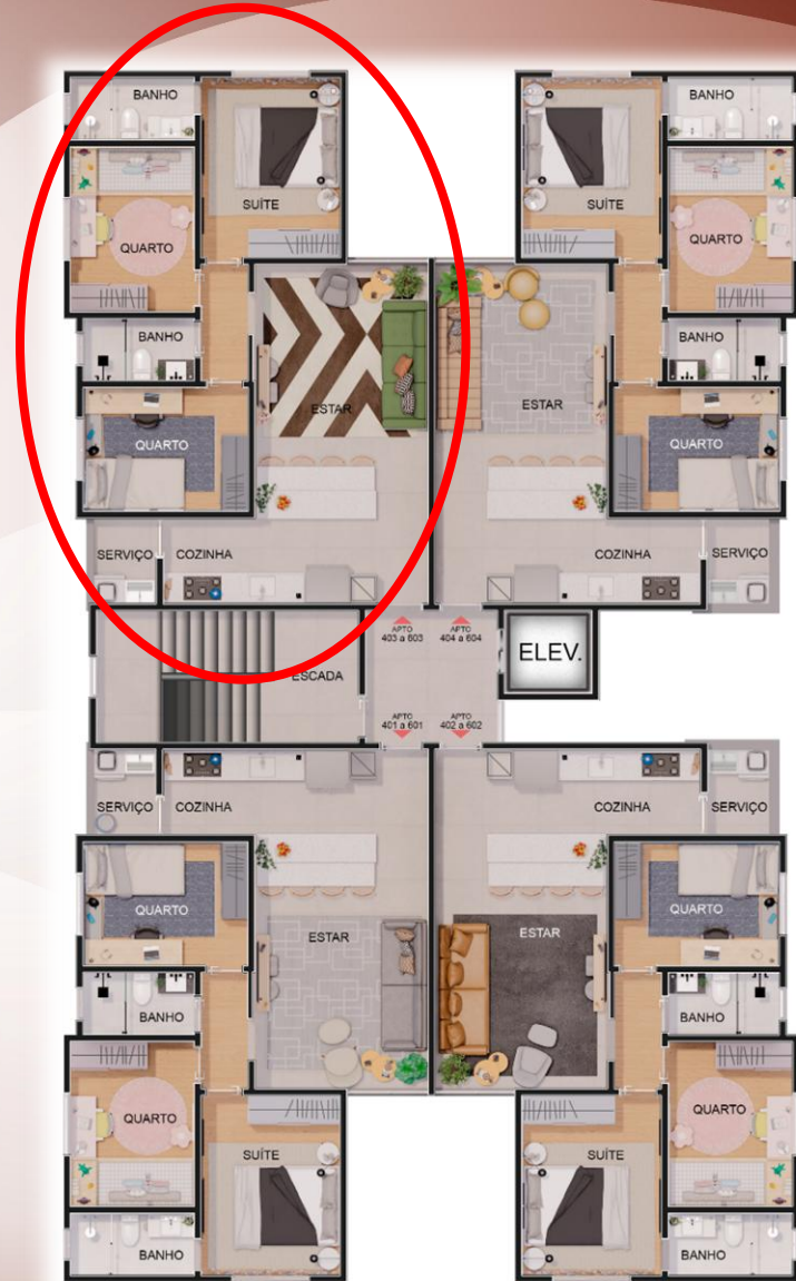
PLANTA 4º a 6º PAVIMENTO - APARTAMENTOS TIPO
